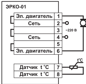
Рис.4 Схема подключения.
