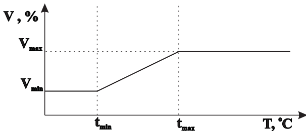
Рис.2 Зависимость скорости вращения вентилятора от температуры. (Профиль №1).
