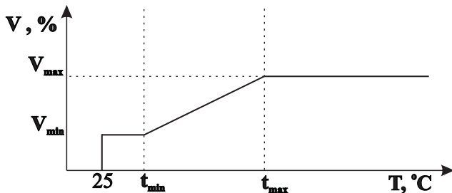
Рис.3 Зависимость скорости вращения вентилятора от температуры (Профиль 2).
