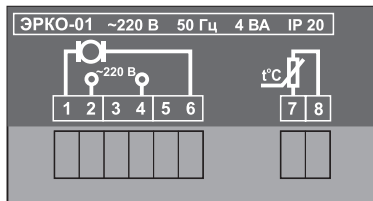
Рис. 5 Вид задней панели ЭРКО-01.
